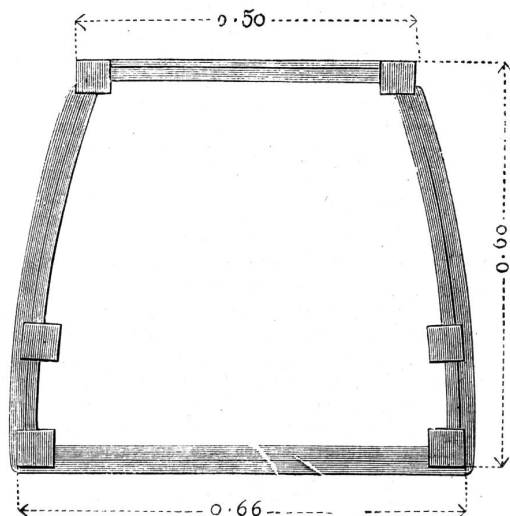
Grundriss.
