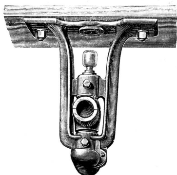
Geschlossenes Hänglager
