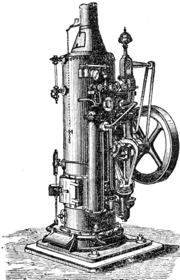
Klein'scher Sparmotor
