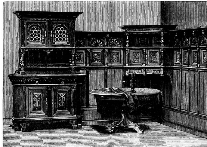
Höhe der Täfelung 1,85 m, Höhe des Buffet 2,20 m, dessen Plattenbreite 1,40 m. Die Füllungen der einzelnen Felder in Holzschnitzerei ausgeführt und unter einander verschieden. Beschläge Schmiedeeisen.
