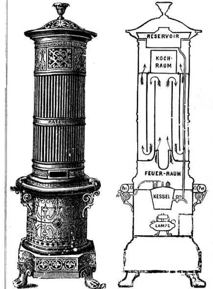
Petroleum-Ofen für Zimmerheizung von Robert Schulz.
