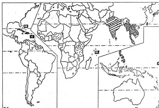
Die bezeichneten Gebiete auf der obestehenden Karte geben an, wo in den letzten Jahren regelmässig (schraffiert) oder gelegentlich (punktiert) Dengue aufgetreten ist. Die Kästchen bedeuten, von Westen nach Osten: 1. Bahamas. 2. Kleine Antillen. 3. Seychellen. 4. Die Inseln der Süde.
