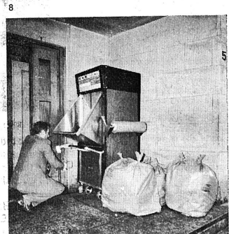
1 Flaschenzertrümmerer der Fa. Kisag AG, Bellach. Durch die Einfüllöffnung wird die Flasche in den Apparat geworfen, der dann in Gang gesetzt wird. Und im darunterstehenden Sack wird der Flaschengrüss für den Abfalltransport gesammelt.
