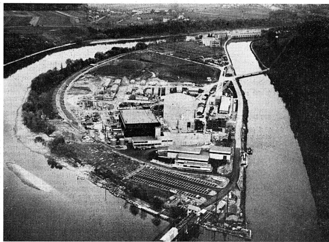
Das zweite Sicherheitsgebäude des Atomkraftwerkes auf der Insel Betznau nimmt Form an. Bereits sind die Fundamente erstellt und gegenwärtig sind die Arbeiten am Schutzmantel in vollem Gang. 1972 soll das Zwillingsatomkraftwerk eine jährliche Energiemenge von 5 Milliarden Kilowattstunden abgeben. Unsere Flugaufnahme zeigt eine Gesamtübersicht über die Insel Betznau mit dem ersten schweizerischen Atomkraftwerk mit Leichtwasserreaktoren. Photopress
