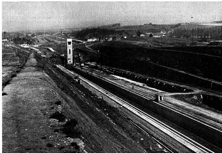
Tremée de rive gauche du plan incliné (partie enterrée).
