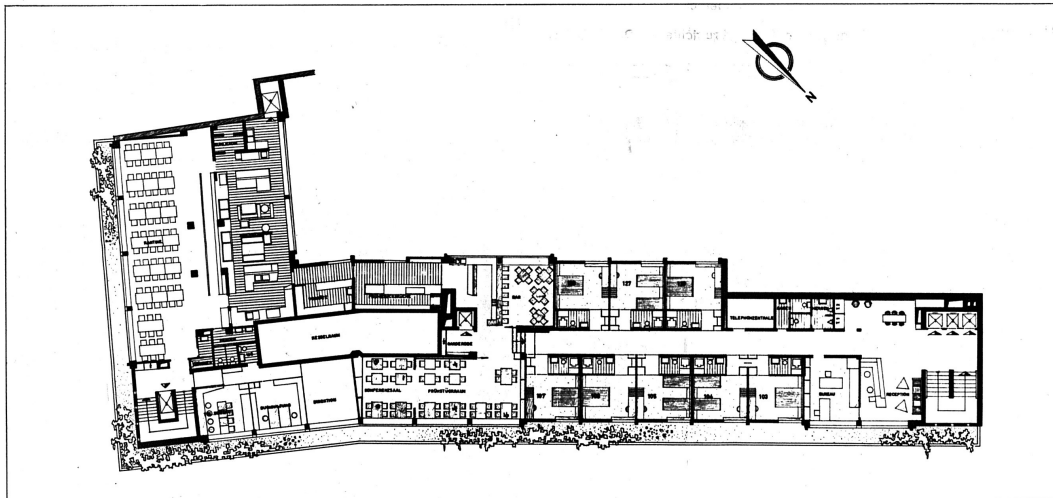
1. Obergeschoss 1:200
