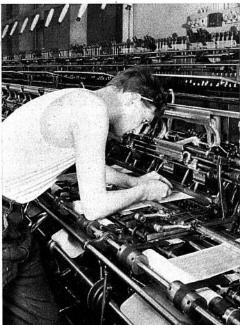
Wirker beim Nadelrichten an der Cotton-Wirkmaschine
