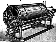
Universal-Doppeltrammel-Dampfwäschmaschine mit verbesserter Dreiecksform und hinterlegtem Vorgelege (D. R. Patent und mehrfachen D. R. G. M.).
