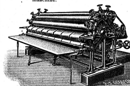
Universal-Dampfmangel- und Plättmaschine mit Essener Umlauf durch mehrfachen D. R. G. M. geschützt.
