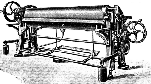
Komplette Wascheinrichtungen. C. Séguin, Constructeur, Mülhausen I. E.
