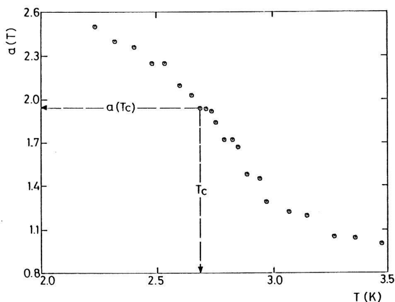
Figure 2 : Variation de l'exposant a(T) avec la température pour l'échantillon décrit figure 1.
