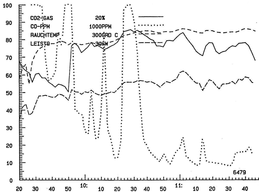
Fig. 3 Verbrennungsqualität - Rauchgastemperatur
