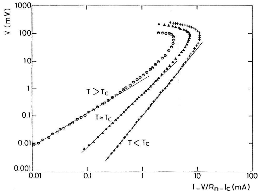
Figure 1 : Caractéristiques expérimentales V(I_S) aux températures 3.072 K, 2.713 K et 2.233 K d'un échantillon de tantale ( R_N = 5.05 \Omega , T_c = 2.69 K). Les valeurs de a(T) sont 1.22, 1.94 et 2.5.
