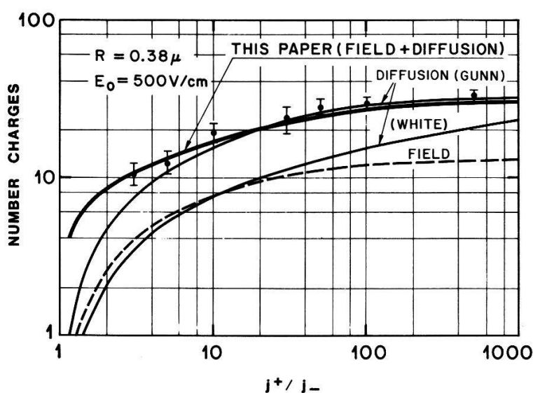
Fig. 4. Vergleich verschiedener Theorien mit gemessener Ladung auf einem Latex-Teilchen mit Radius = 0,38 \mu , als Funktion des Verhältnisses j^+/j^- . Die Aufladezeit betrug t = 0.2 s und n_0 = 6 \cdot 10^7 \text{ cm}^{-3} .
