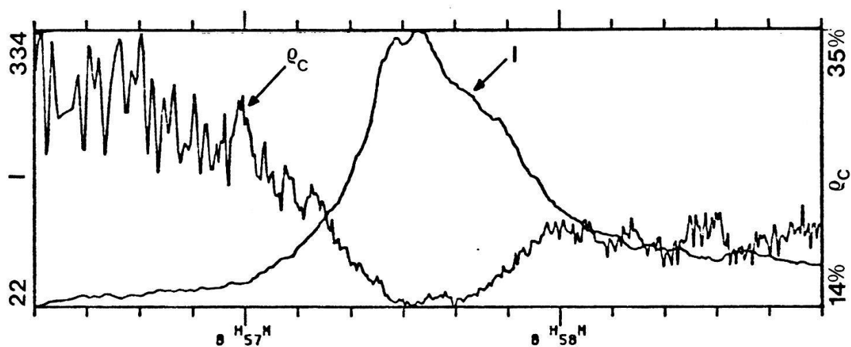
Fig. 1: 26. April 1984. Intensität I ( 10^{-22} \text{ W m}^{-2} \text{ Hz}^{-1} ) und Polarisationsgrad \rho_C bei 11,8 GHz
