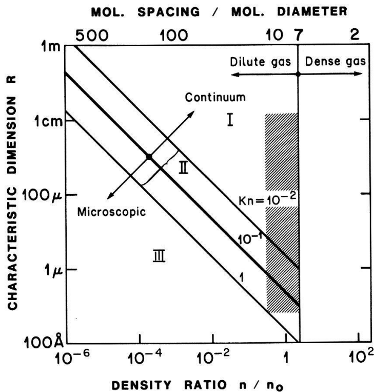
Fig. 2. Die drei Aufladungsbereiche. n_0 = 2.4 \cdot 10^{19} \text{ cm}^{-3} .
