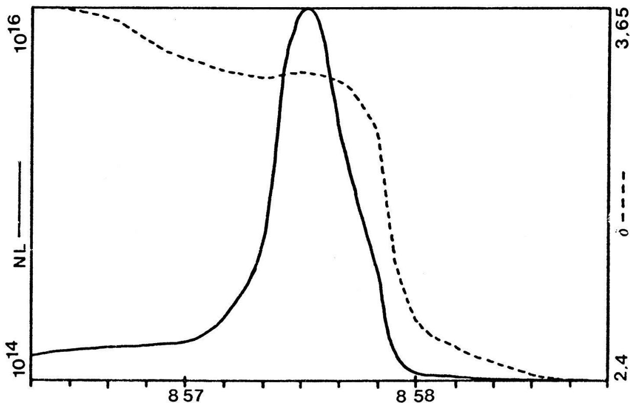
Fig. 3: Zeitlicher Verlauf von column density NL ( \text{cm}^{-2} ) und Spektralindex \delta
