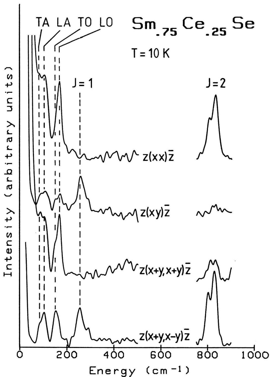
Fig. 2: Polarisierete Ramanspektren von \text{Sm}_{.75}\text{Ce}_{.25}\text{Se}
