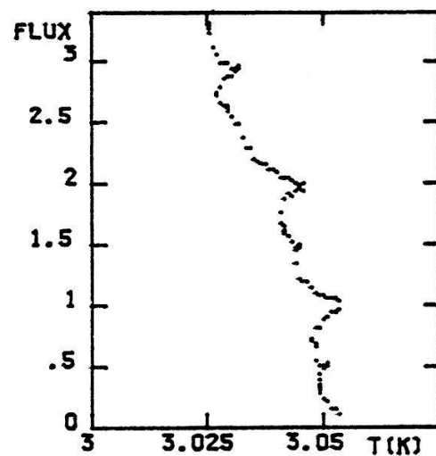
Figure 2b : Ligne de transition supraconductrice.
