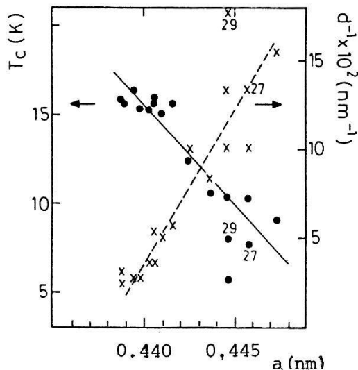
Fig. 1 : Variation de la température critique T_c et de l'inverse de la taille des grains d^{-1} en fonction du paramètre de maille a .
