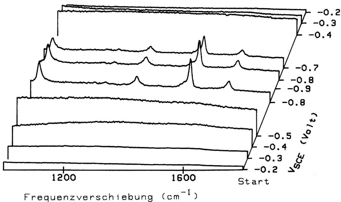
Fig. 1: Ramanspektren von MV^+ auf einer "glatten" Silberoberfläche als Funktion des Elektrodenpotentials.
