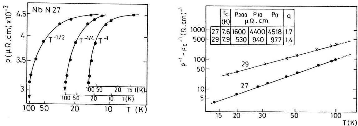
Fig.3 : Lois du type \rho(T) \propto \exp(T_0/T)^n pour n = 1 ; n = 1/2 ; n = 1/4 .
