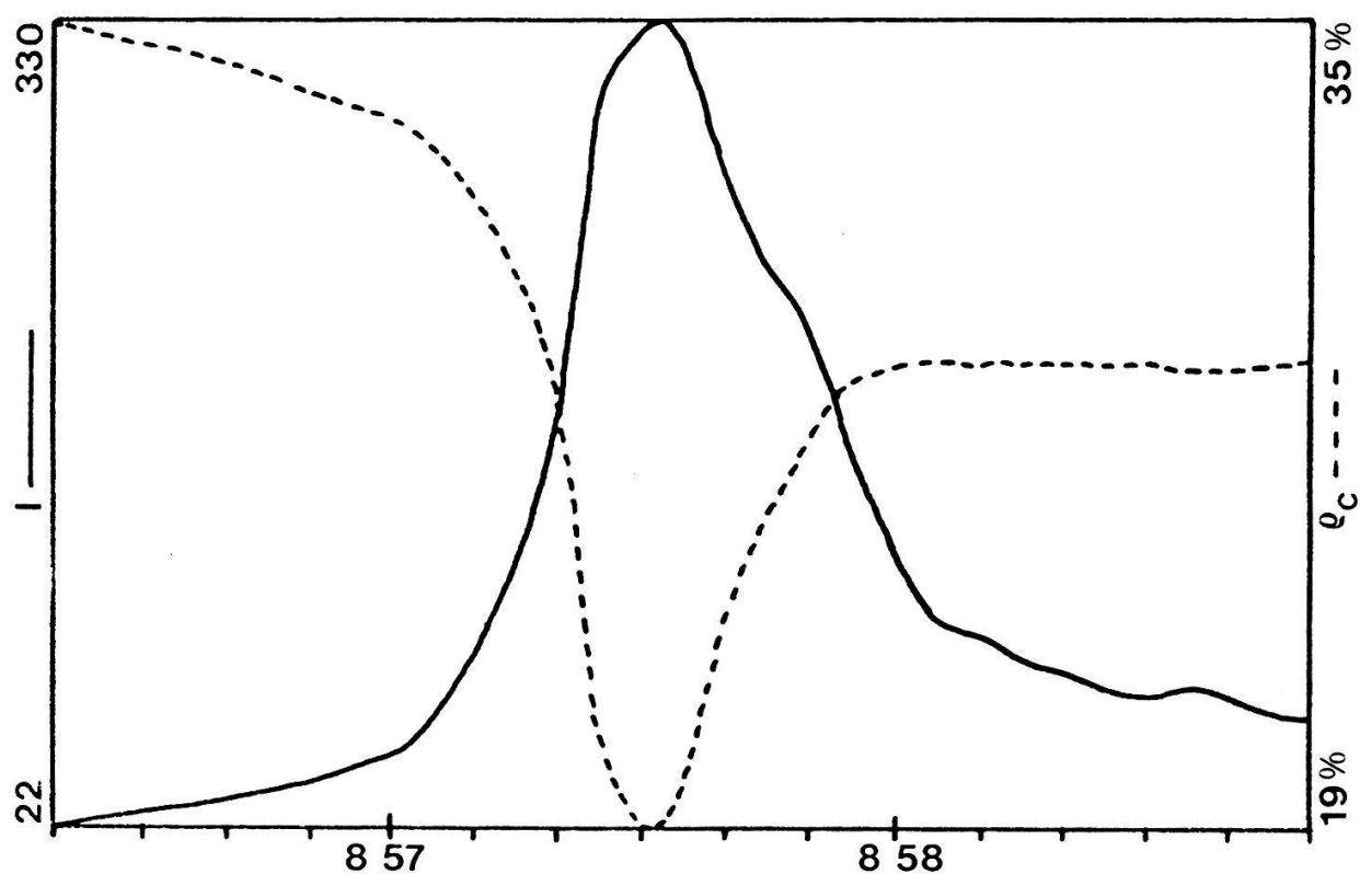
Fig. 2: Simulierter Zeitverlauf von Intensität I und Polarisationsgrad \rho_C des beobachteten Bursts (Fig. 1). Beobachtungswinkel: 75^\circ
