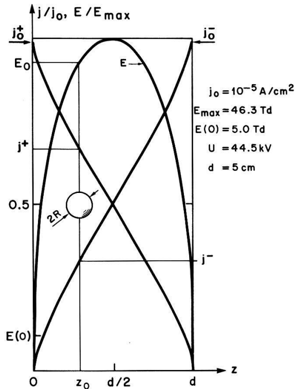
Fig. 1. Das elektrische Feld und die Ionenströme in einer eindimensionalen Entladungsstrecke. Das Teilchen mit dem Radius R befindet sich an der Stelle z_0 .
