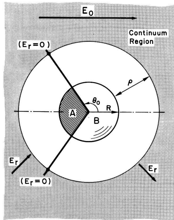
Fig. 3. Die Randzone um das aufgeladene Teilchen herum.
