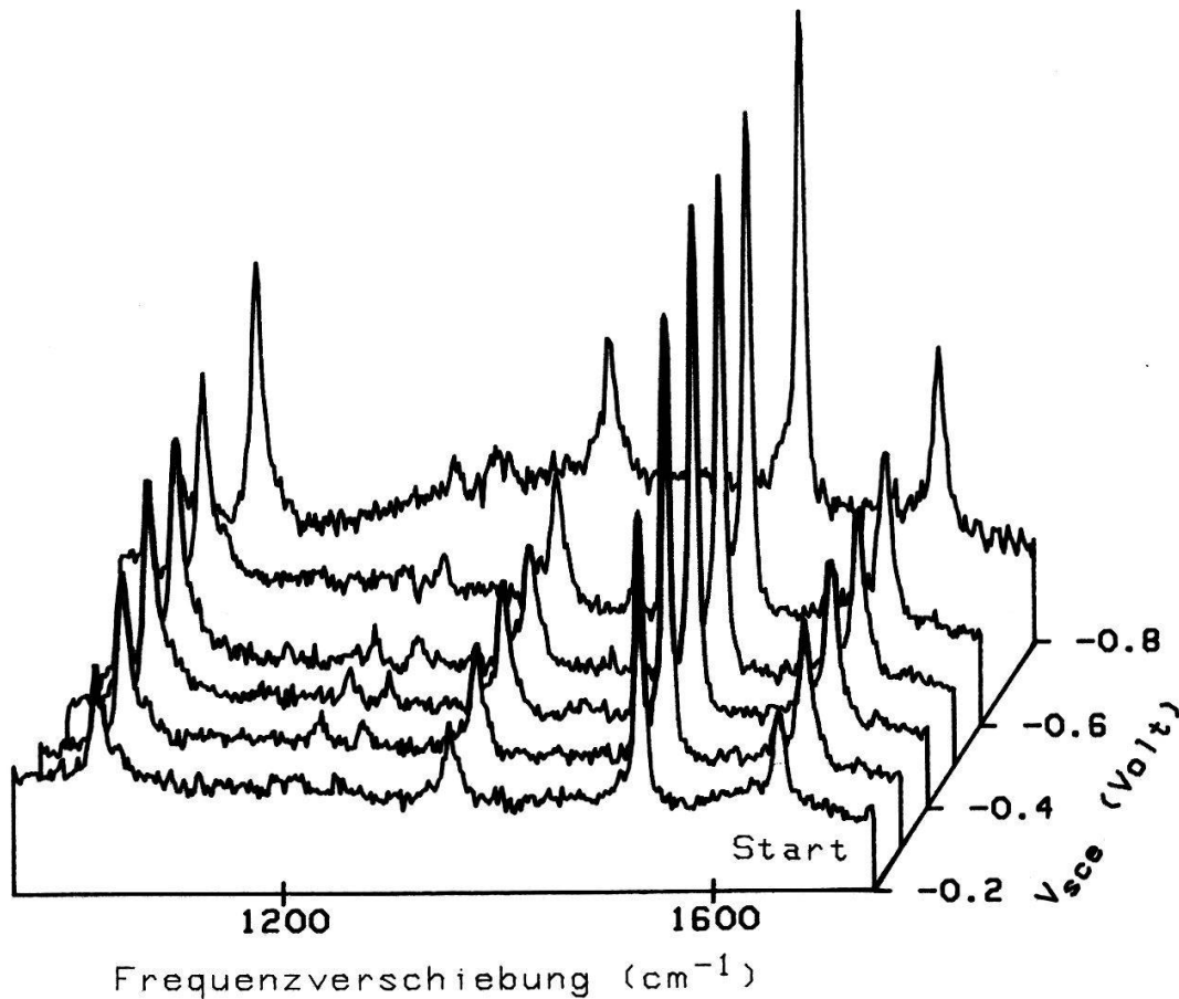
Fig. 3: Ramanspektren von MV^+ auf einer \beta\text{-ZnP}_2 Elektrode als Funktion des Elektrodenpotentials.
