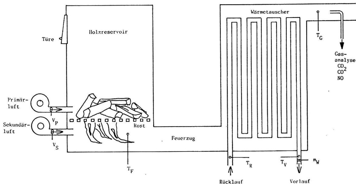
Fig. 1 Schema des untersuchten Versuchsofens
