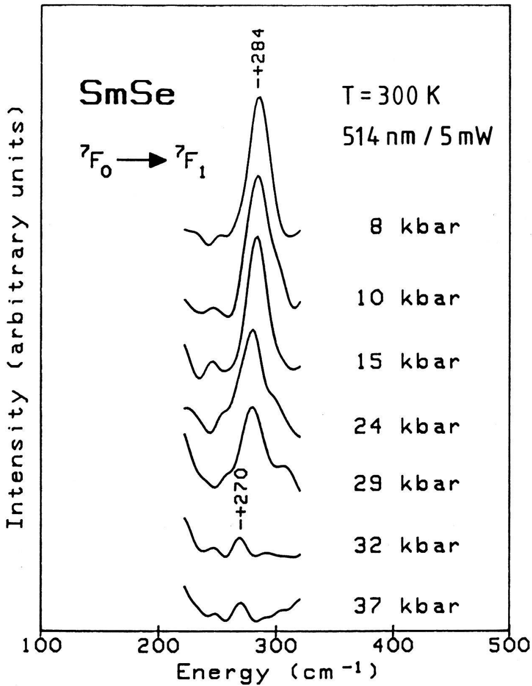
Fig. 1: Ramanspektrum des {}^7F_J - Zustandes in SmSe unter Hochdruck. Die kleinen Strukturen auf beiden Seiten und der Peak bei 270 \text{ cm}^{-1} stammen vom Druckübertragungsmedium
