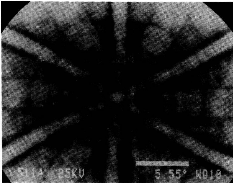
Fig. 2. REM-Channeling Diagramm von epitaktischem CdTe auf (\text{Ba,Ca})\text{F}_2/\text{Si}(111) .
