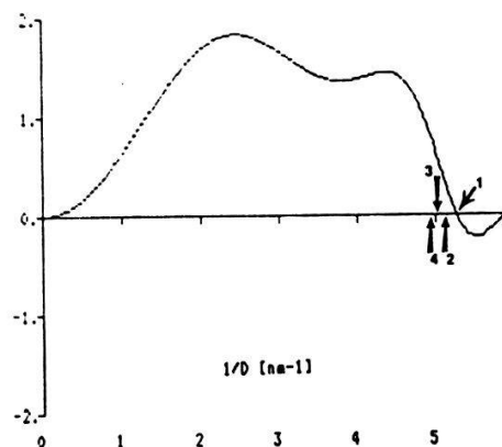
Fig. 1 : Fonction de transfert C_s = 1.1 \text{ mm} (1), 1.15 (2), 1.2 (3), 1.3 (4); tension 300 kV
