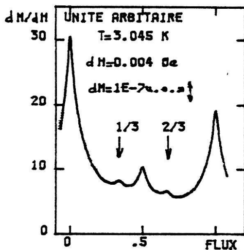
Figure 2a : Oscillations de dM/dH en fonction du champ magnétique appliqué normalisé au quantum de flux par boucle.
