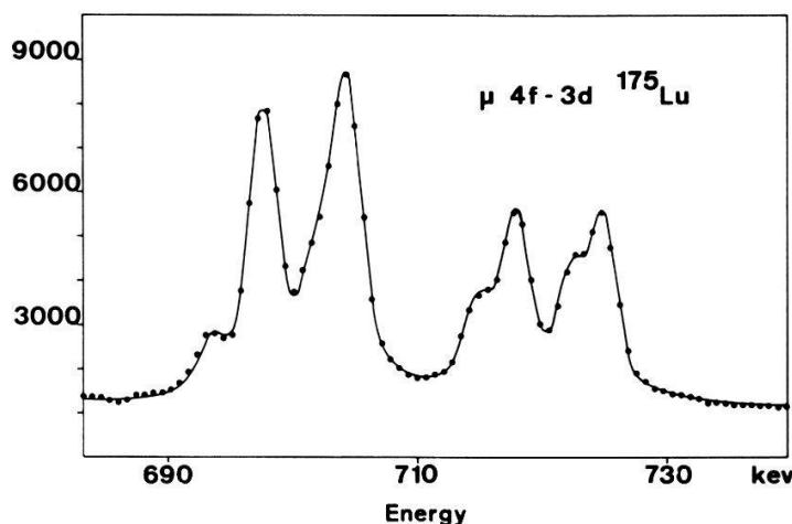
Figur 1 Myonischer 4f-3d Röntgenübergang in ^{175}\text{Lu} .
