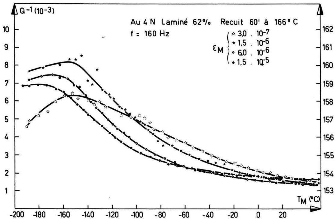
Figure 2 Frottement intérieur mesuré en fonction de la température pour quatre amplitudes de vibration différentes, métal recristallisé après fort écrouissage (62%).
