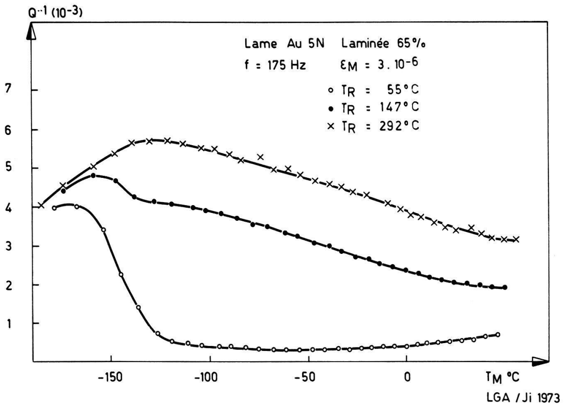
Figure 1 Frottement intérieur dans l'or écroui, en cours de recristallisation ( T_R = 147^{\circ}\text{C} ) et recristallisé ( 292^{\circ}\text{C} ) mesuré en fonction de la température.
