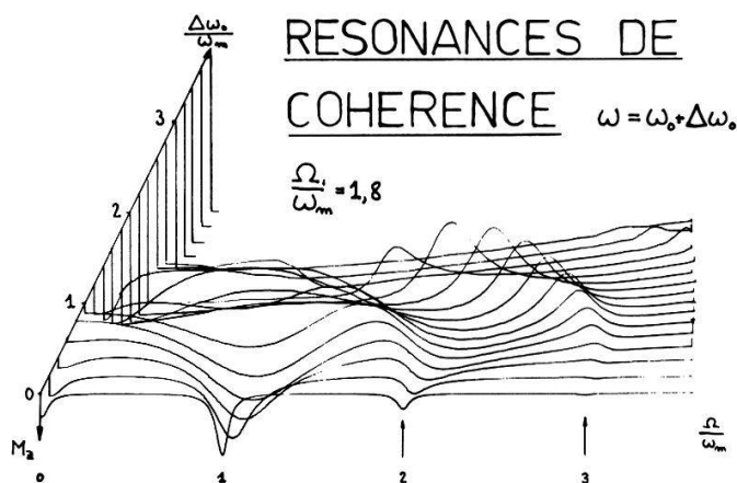
Figure 1 Résonances de cohérence et à quanta multiples (simulation analogique des équations de Bloch).
