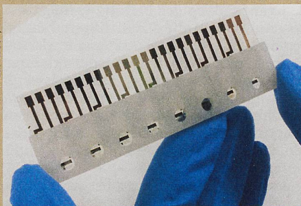
Acht Nöpfchen für elektrochemische Messungen.
