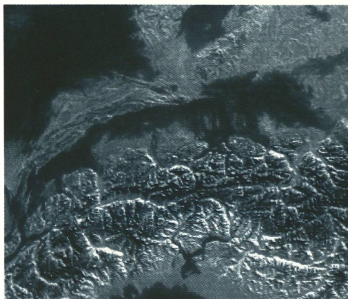
Diese Satellitenbilder der Schweiz um Mittag weisen die idealen Bedingungen für die Ausarbeitung neuer Techniken zur Bildinterpretation auf. Links: 9. Jan. 1989, kein Wölkchen, dafür eine dicke Nebeldecke über Nordeuropa, dem Mittelland, dem Lago Maggiore und dem Potal. Rechts: 27. März 1989, strahlende Sonne ohne Wolken und Nebel. (Photos: NOAA 11)
