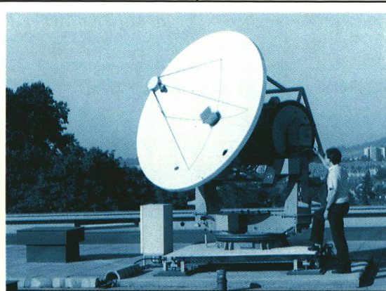
Cette antenne parabolique, pilotée par ordinateur, pivote sur deux axes. Elle a été construite pour suivre automatiquement les trajectoires des satellites météorologiques et recueillir ainsi leurs informations. (Photo: Uni. de Berne)
