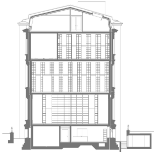
^Querschnitt.
