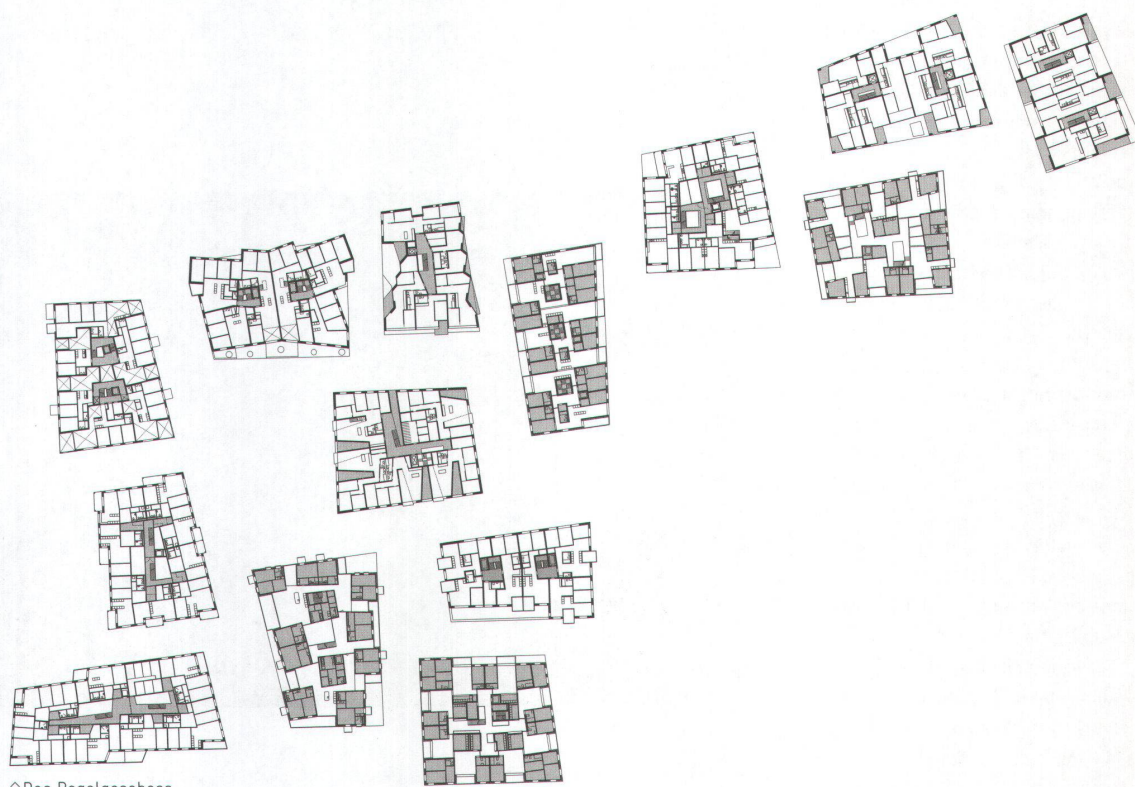
^ Das Regelgeschoss.
