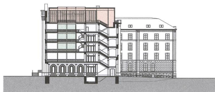
Querschnitt
