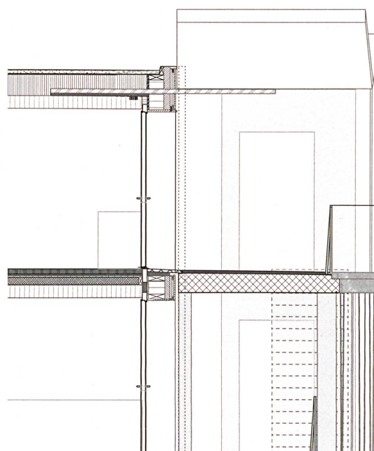
Detail Fassade.
