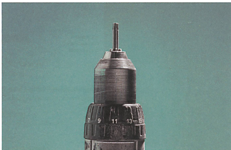
Bohrfutter mit Torx-Einsatz. | Mandrin avec insert Torx. | Mandrino portapunta con inserto Torx.
