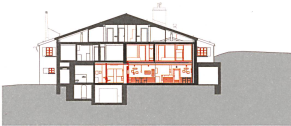
Ospizio Bernina, Schnitt.
