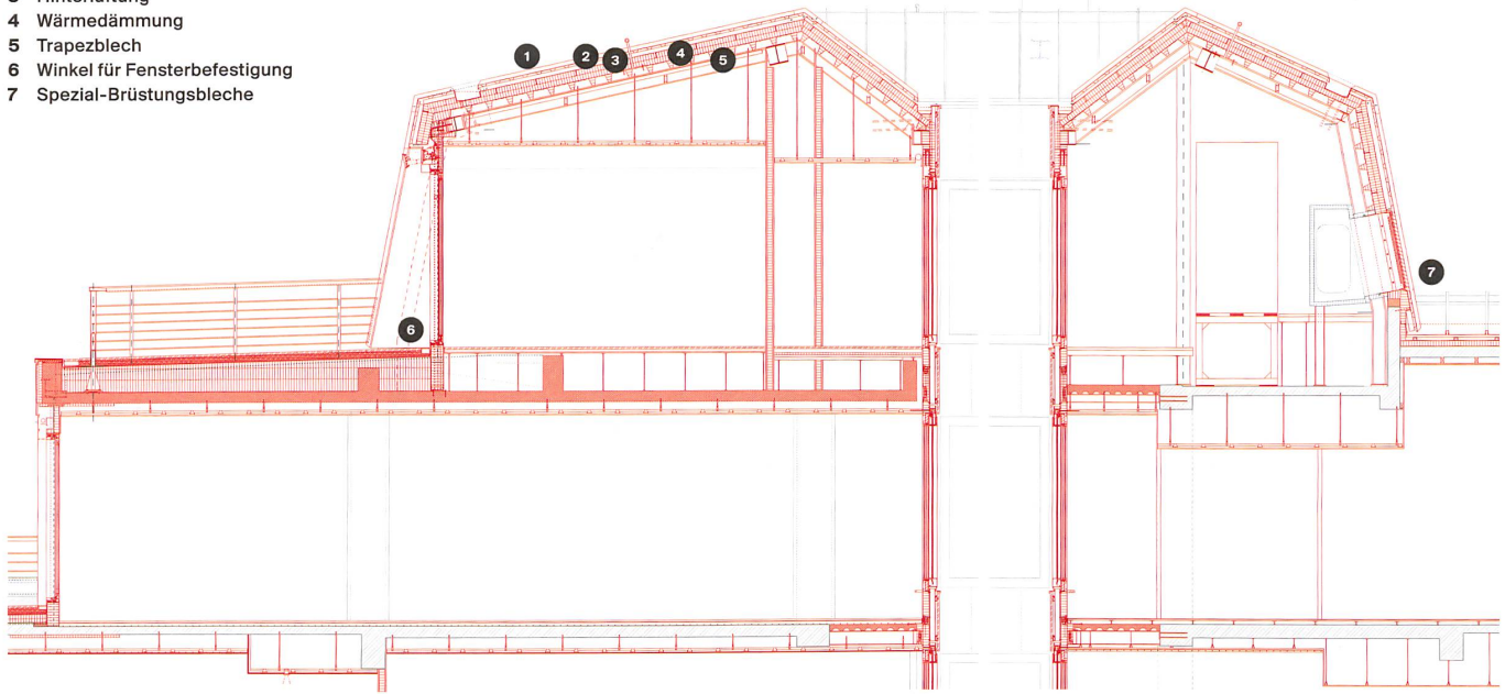
Querschnitt 4.-6. Obergeschoss: Eine grosse Herausforderung waren die Abläufe, die in die Unterkonstruktion integriert wurden.
