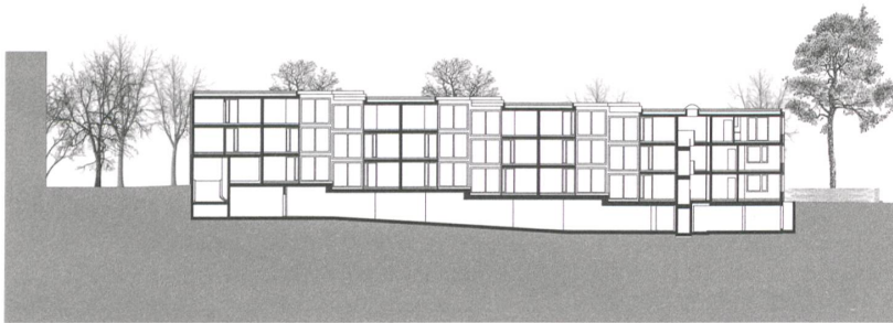
Längsschnitt
