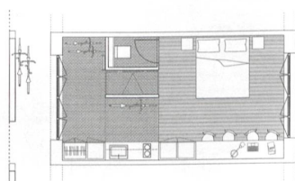
Schnitt und Grundriss eines Sportzimmers.
