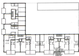
Regelgeschoss
