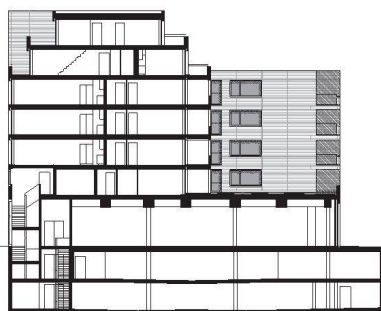
^2_Querschnitt
