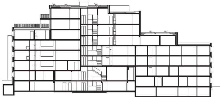
^ Längsschnitt: Das Treppenhaus im neuen Mittelteil verbindet die um ein halbes Geschoss versetzten Altbauten.
