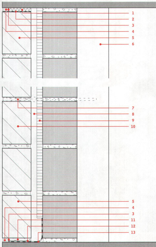
Fassadendetail Kopf- und Fusspunkt
