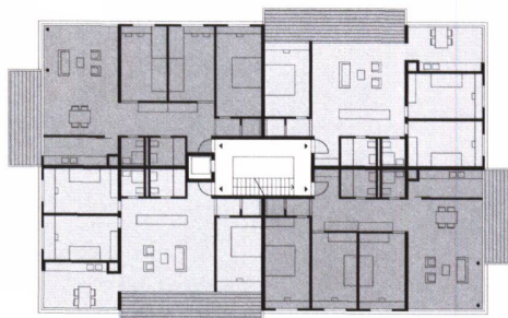
Normgeschoss
