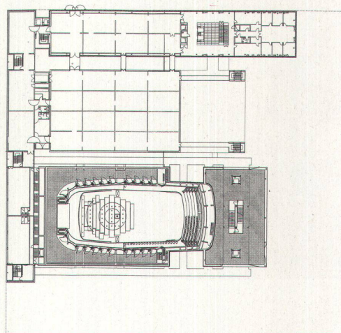
Grundriss vierter Stock: Das Museum verteilt sich auf zwei Trakte, unten der Luftraum des Konzertsaaes
