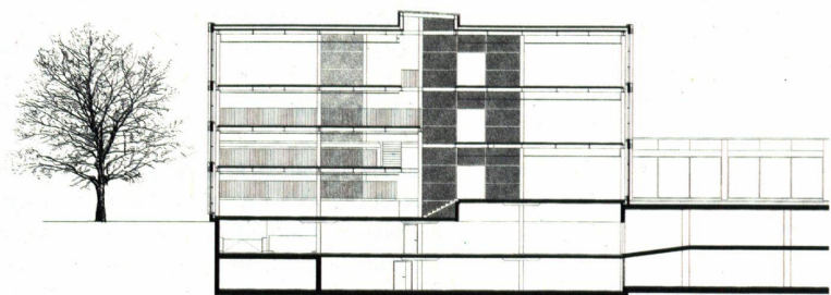
Schnitt des Annexbaus. Die Architekten haben den Bau aufgestockt, die Treppen, Licht- und Lüftungsschächte zu Service-Türmen gefasst
