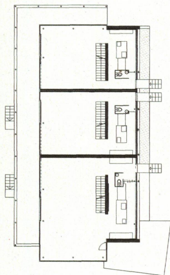
Grundriss Erdgeschoss
