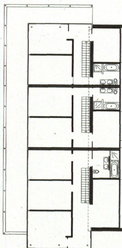
Grundriss Obergeschoss
