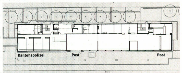
Erdgeschoss
