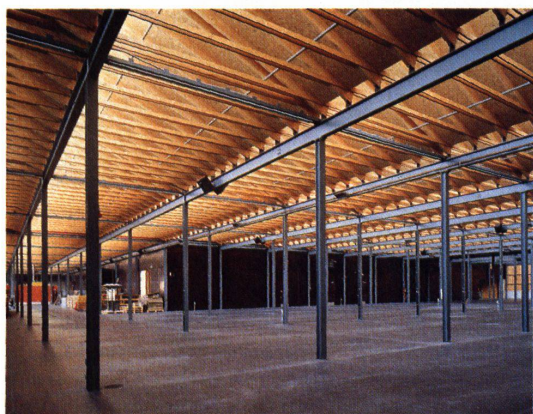
Die Viehmarkthalle ist eine einfache Stahlstützenkonstruktion, auf der ein Holzsheddach liegt
