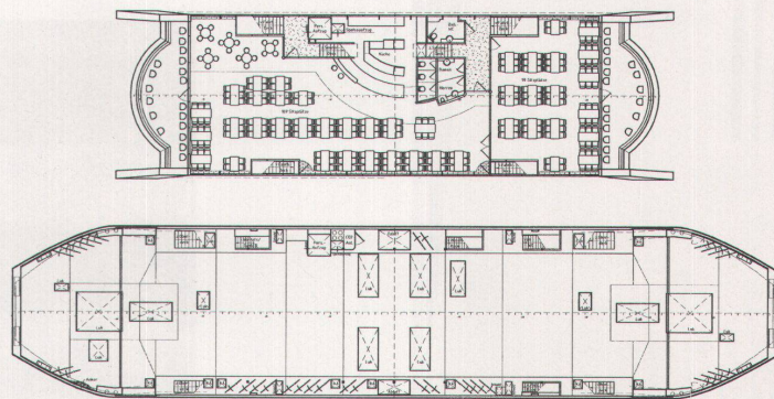
Grundrisse: Fahrbahndeck und Oberdeck
