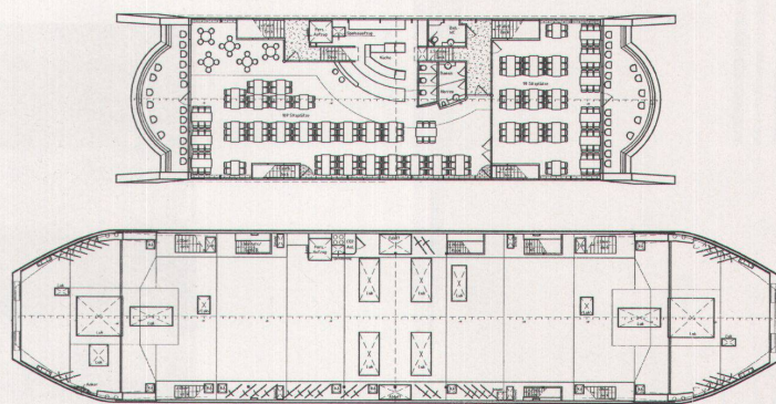
Grundrisse: Fahrbahndeck und Oberdeck
