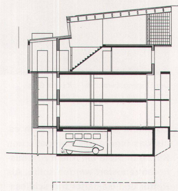
Querschnitt
