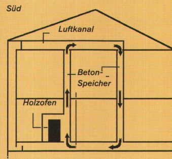
Schema der Luftführung bei Ofenbetrieb
