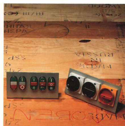
Produkt: Multifunktionsstaste DM 3 und Haupt-Notausschalter L2 (rechts) Design: Fernand Hofer, Sprecher + Schuh Werkdesign, Aarau Hersteller: Sprecher + Schuh, Aarau
