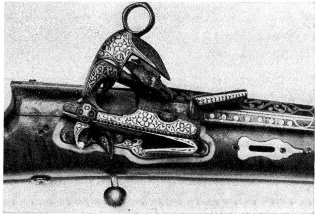
Fig. 147. Schnapphahnschloss des Gewehres 299.
