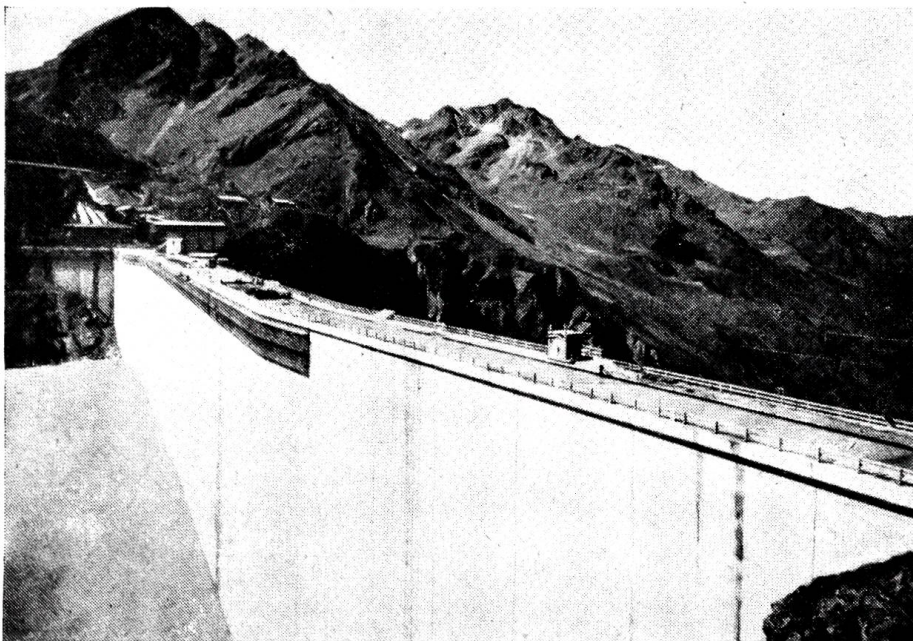
Die höchste Staumauer Europas fertig betoniert. Die Staumauer der Grande-Dixence: Höhe 285 m, Kronenlänge 748 m.
