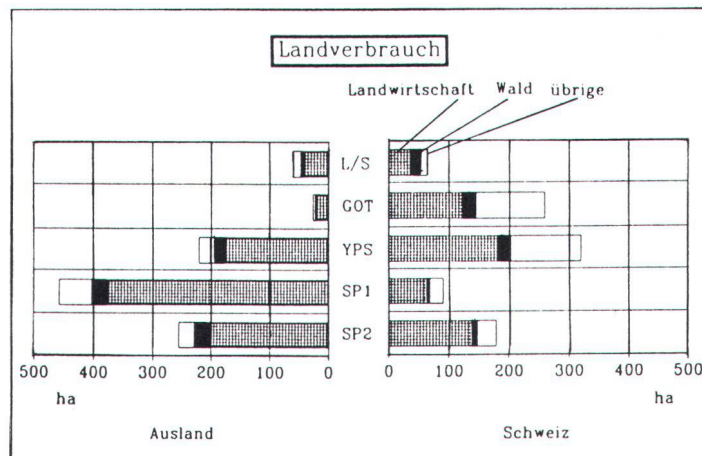
NEAT-bedingter Landverbrauch für Neu- und Ausbaustrecken in der Schweiz und im Ausland. Danach schneidet die Lötschberg-Simplonlinie am besten ab, gefolgt von der Variante Splügen I. Empiètement dans le terrain de la NLFA, pour des tronçons nouveaux et des extensions, en Suisse et à l'étranger. On voit que c'est la solution Loetschberg-Simplon la meilleure, suivie du projet Splügen I.
