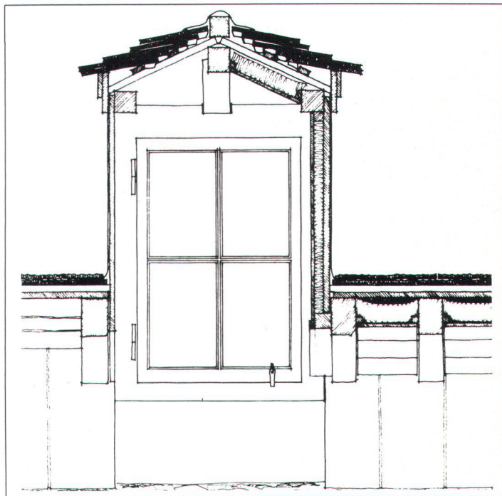
Coupe transversale, vue de l'intérieur: à gauche l'état actuel, à droite un projet d'isolation (illustration Baertschi).
