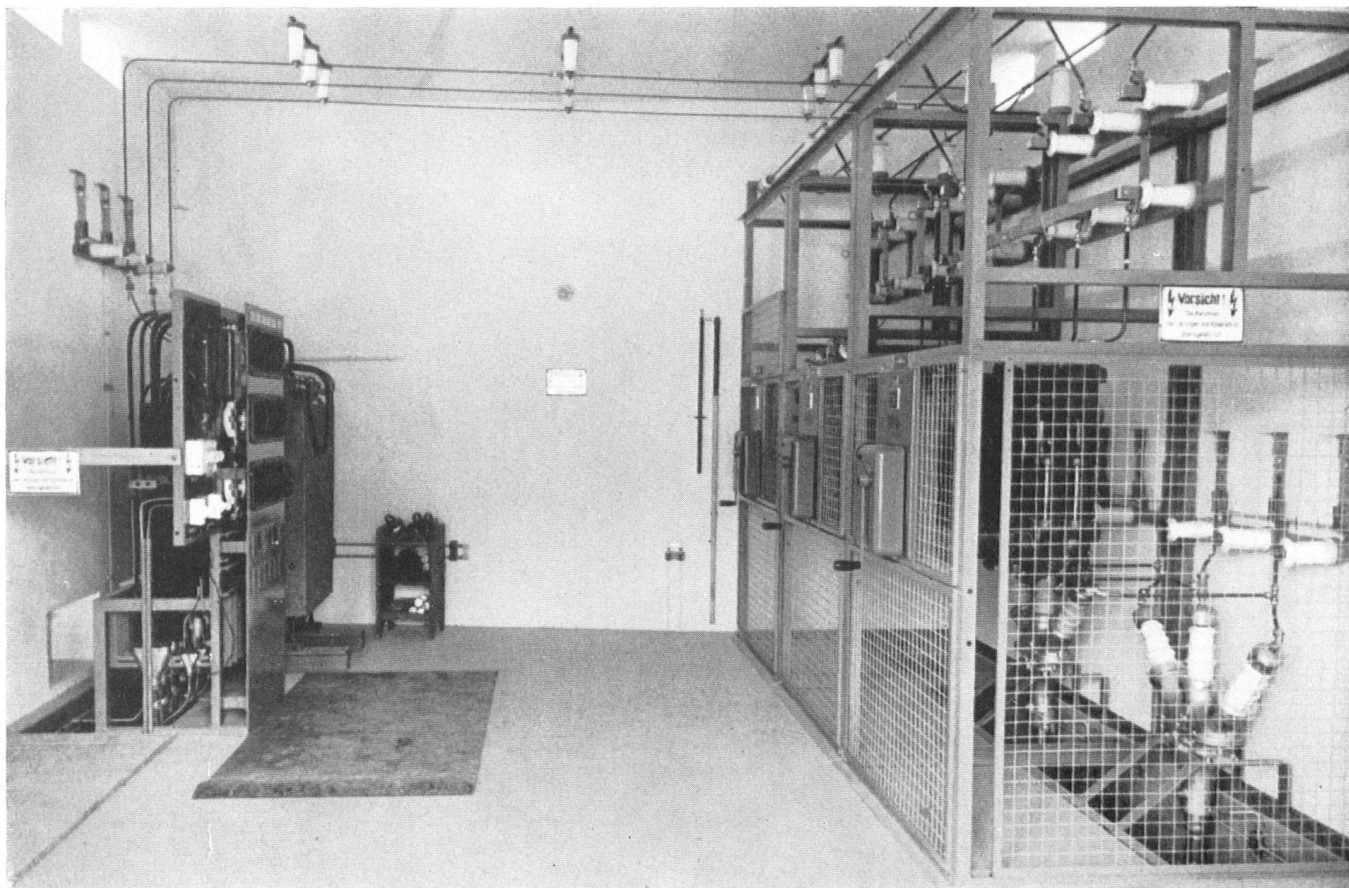
Was in den An- und Zwischenbauten heute verborgen wird: Inneres der Transformatorstation Adliswil, siehe Vorderseite. Rechts die Hochspannungsfelder, links der Transformator und davor die Niederspannungs-Verteilung.
