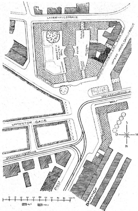
Abb. 2. Projekt der Architekten Rittmeyer und Furrer für die Umgestaltung des Bahnhofplatzes und des Archquartiers: Schliessen des Platzes durch zusammenhängende Baukörper, Abschluss der Stadthausstrasse und der Untergasse. Statt der Archstrasse: hohe Durchfahrten in der den Platz beherrschenden Gebäudefront; hofartige Ausbildung des Strassenstückes zwischen den Durchfahrten, bessere Einmündung der untern Vogelsangstrasse in den Platz. — Fig. 2. Projet des architectes Rittmeyer et Furrer pour la transformation de la place de la Gare et du quartier d'Arch: la place sera encinte d'une série de bâtiments formant un tout compact; d'autres bâtiments serviront d'arrière-plan monumental à la perspective des deux rues: Untergasse et Stadthausgasse. La rue projetée «Archstrasse» sera remplacée par de hauts passages, accessibles aux voitures, percés dans l'enceinte de bâtiments dominant la place; on donnera à l'espace où débouchent les passages le caractère d'une grande cour; l'entrée de la Untere Vogelsangstrasse sur la place sera corrigée.
