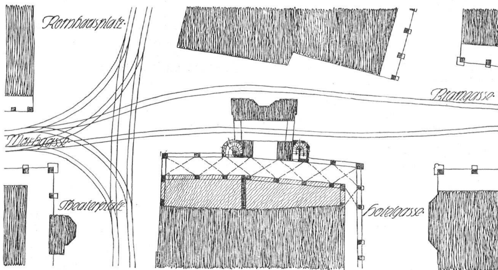
Abb. 26. Situation zum Projekte von Architekt K. InderMühle. Es wird eine erhebliche Verkehrs-erleichterung geschaffen, und das Stadtbild eher bereichert als geschädigt. (Vergl. Abb. 23.) – Fig. 26. Plan de situation du projet de l'architecte InderMühle. La circulation est considérablement facilitée, et l'aspect général y gagne plus qu'il n'y perd.
