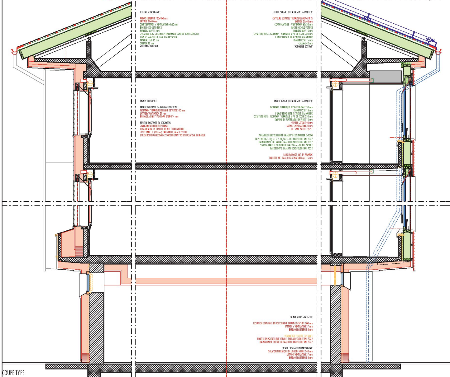
COUPE TYPE
