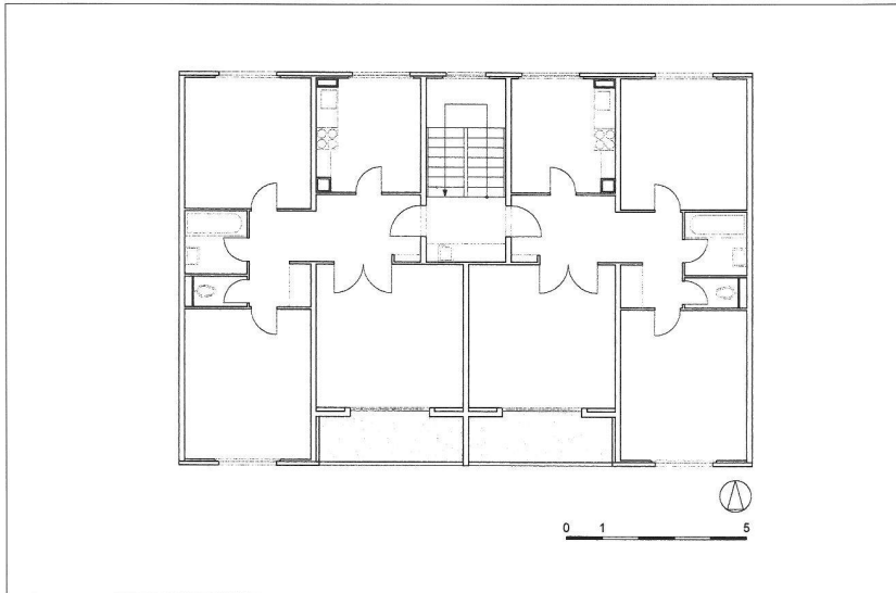
Vetter & Vouga, square de Bellevaux - Pavement, plan de l'étage type de l'immeuble du bas et vue de la façade
