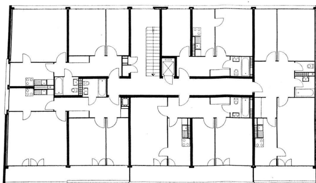
Plan, échelle 1 : 300.
