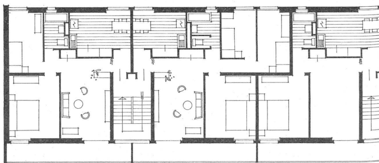
Plan 1 : 300.
