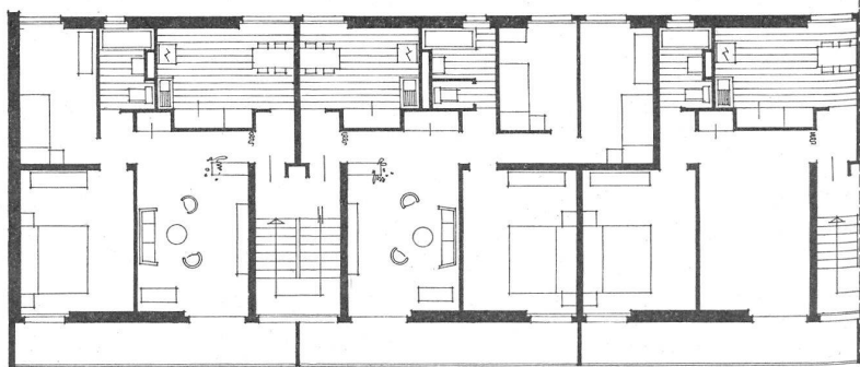
Plan 1 : 300.
